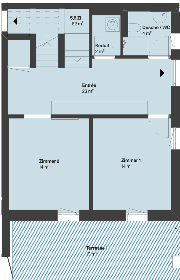
Erdgeschoss
