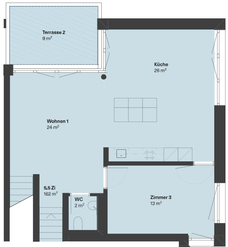
Obergeschoss
