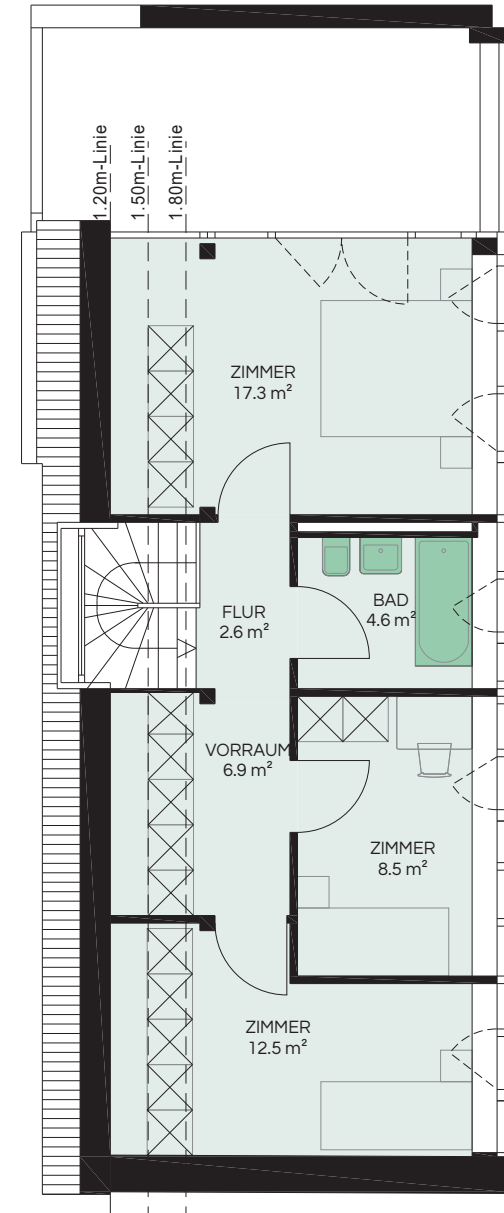
1. OBERGESCHOSS
