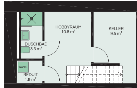
UNTERGESCHOSS
