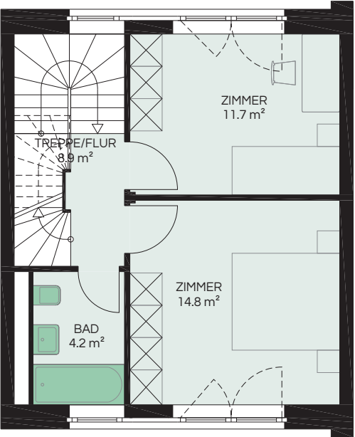
1. OBERGESCHOSS
