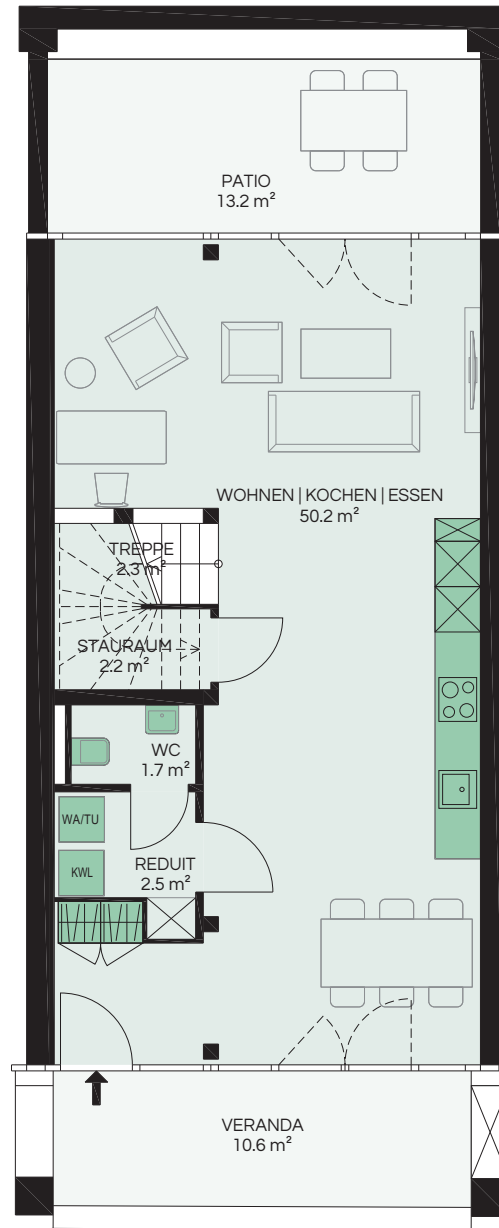
ERDGESCHOSS
