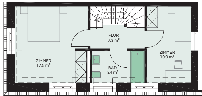
1. OBERGESCHOSS
