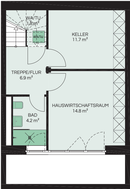
UNTERGESCHOSS
