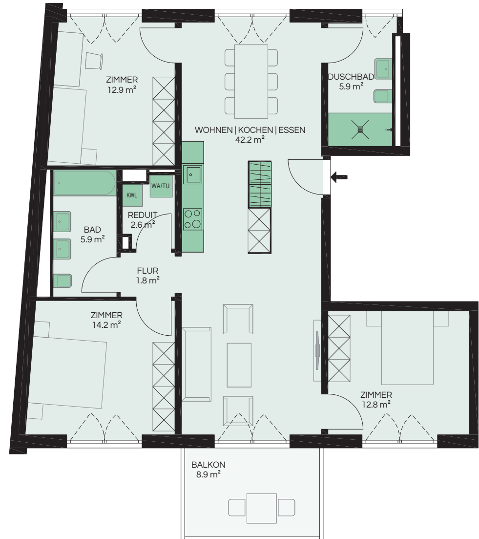
1.OBERGESCHOSS
