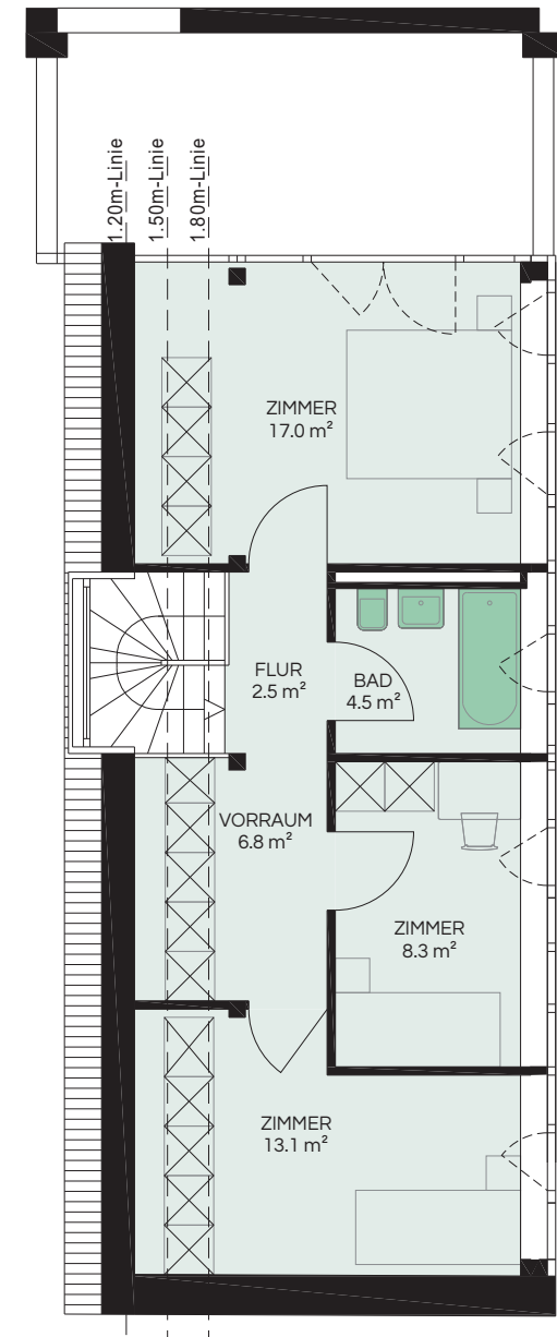
1. OBERGESCHOSS
