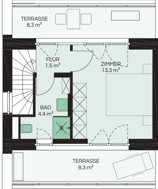
DACHGESCHOSS
