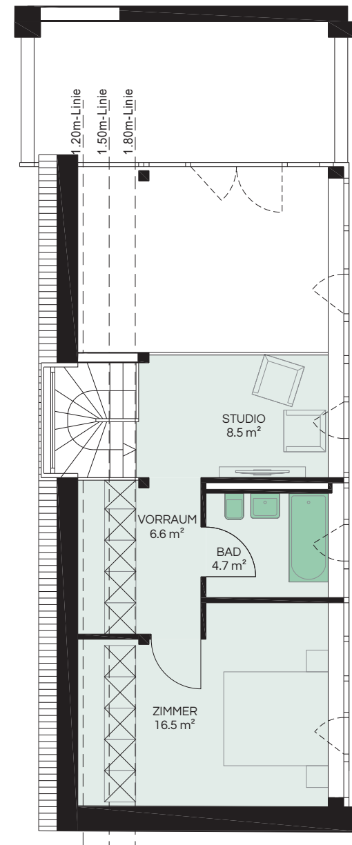
1. OBERGESCHOSS
