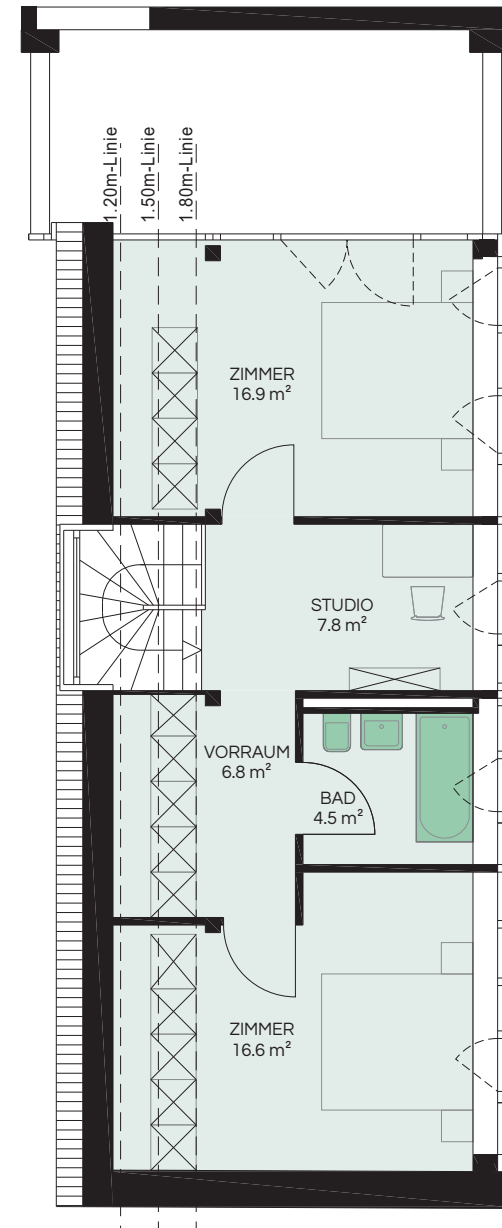
1. OBERGESCHOSS
