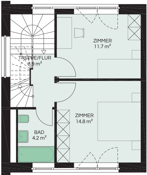
1. OBERGESCHOSS
