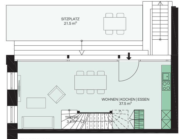
ERDGESCHOSS
