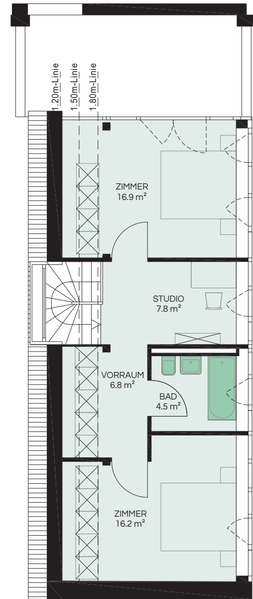
1. OBERGESCHOSS
