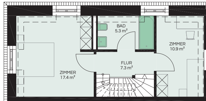
1. OBERGESCHOSS
