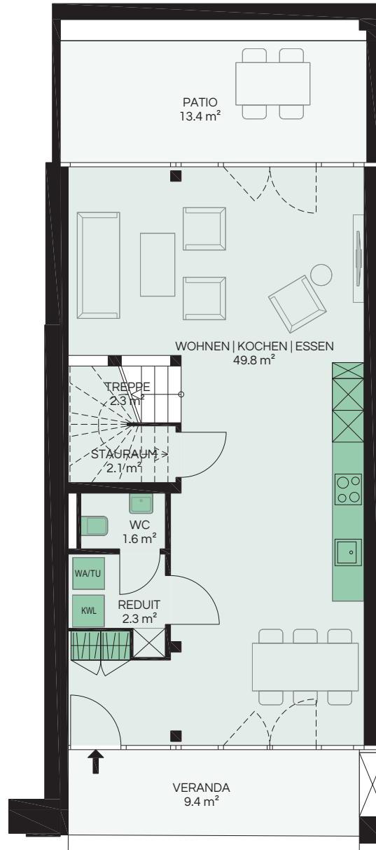
ERDGESCHOSS
