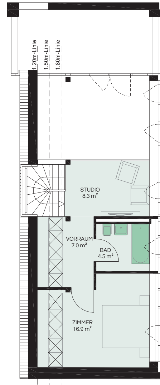
1. OBERGESCHOSS
