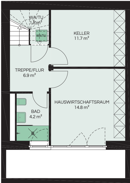
UNTERGESCHOSS
