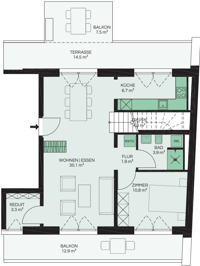
1.DACHGESCHOSS
