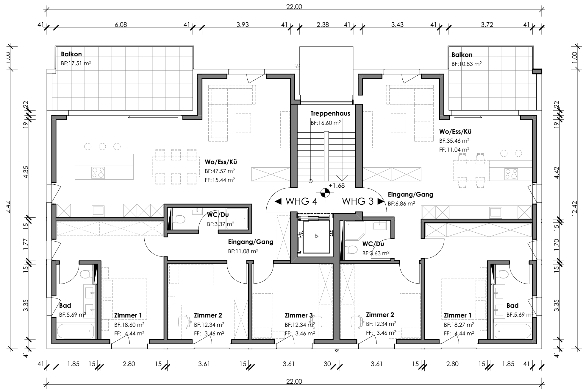
OBERGESCHOSS HAUS WEST
