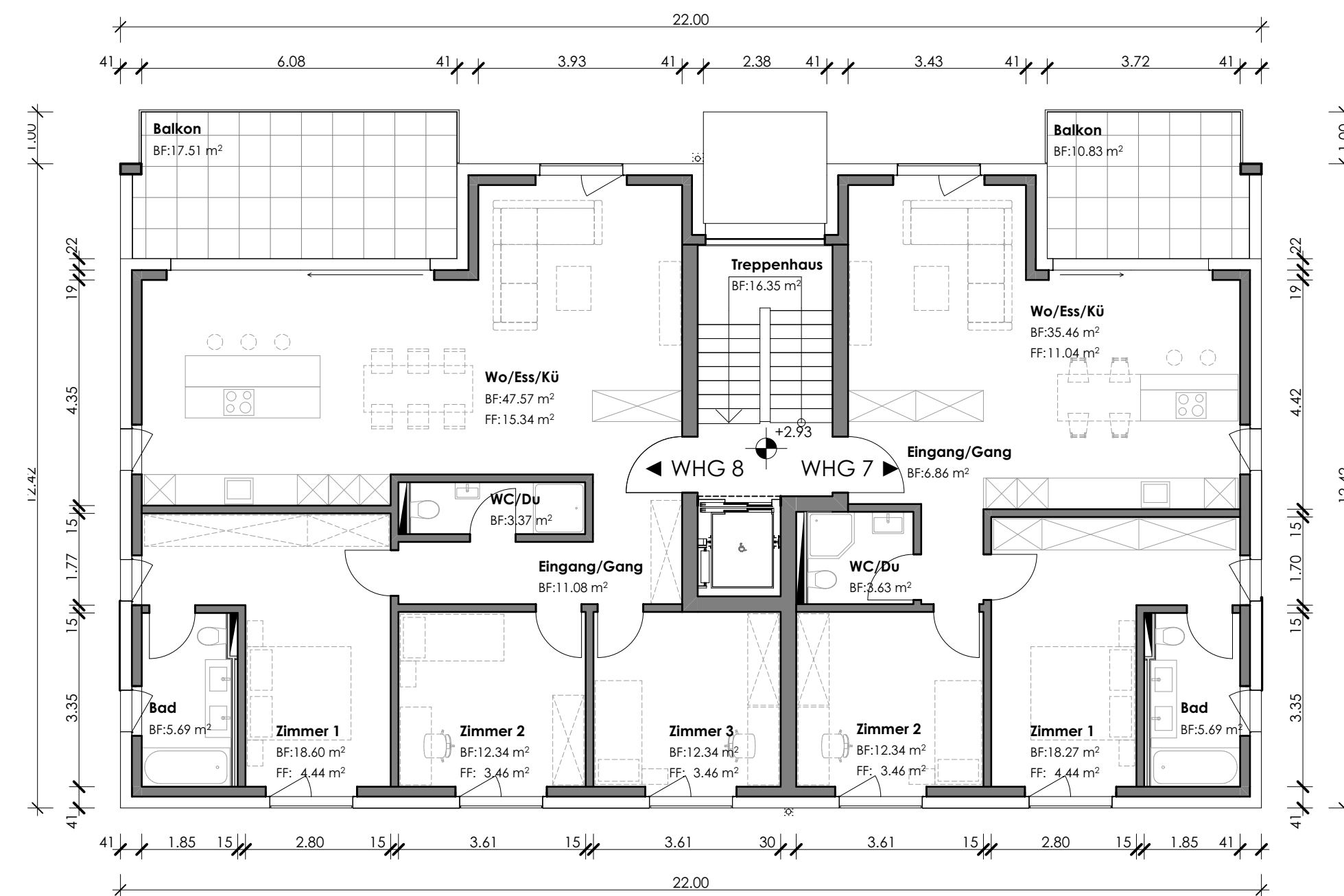
OBERGESCHOSS HAUS OST
